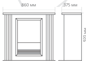
Габаритные размеры:
