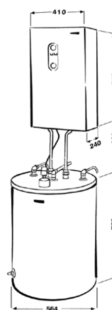
Габаритные и присоединительные размеры SCAT 15K + B120S
